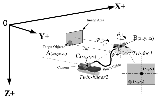
Fig. 1 AUV coordinates
