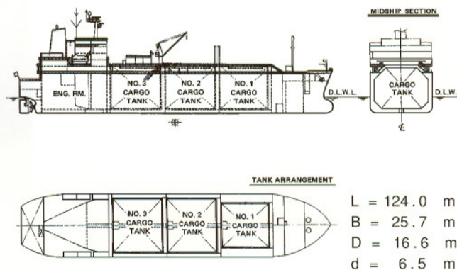
Fig. 1 General arrangement of 18,800 M 3 LNG carrier
